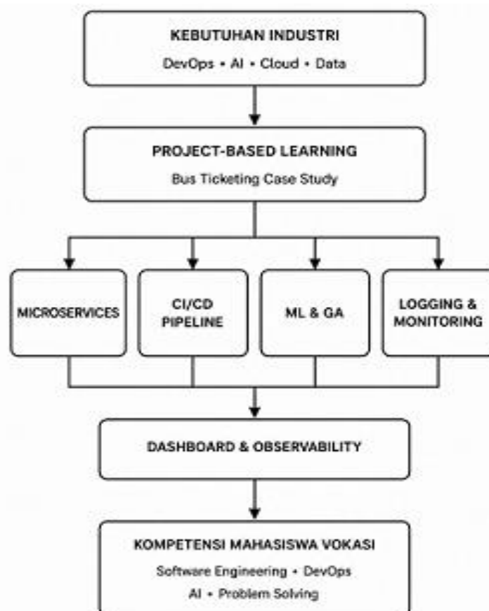
Gambar 1. Kerangka pembelajaran DevOps berbasis industri untuk pengembangan kompetensi mahasiswa vokasi
