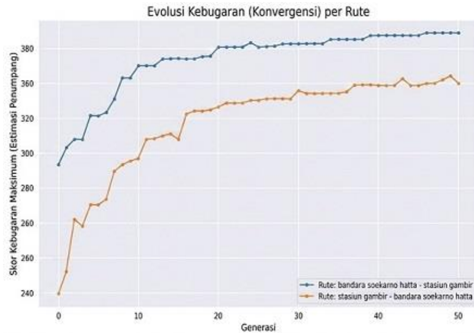
Gambar 7(a). Konvergensi GA
