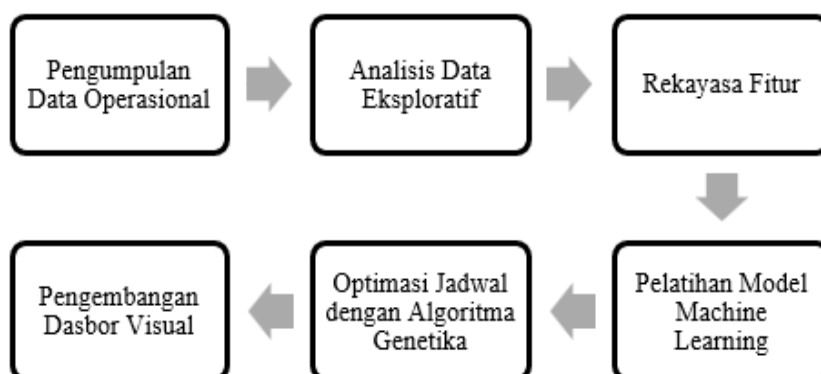
Gambar 2. Metode penelitian untuk modul optimasi jadwal berbasis ML-GA
